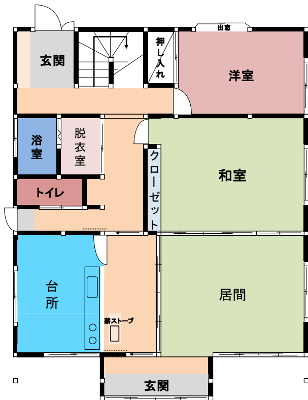
1階平面図
