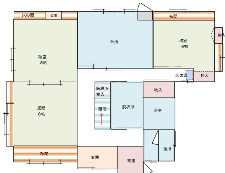
1階平面図
