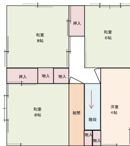
2階平面図
