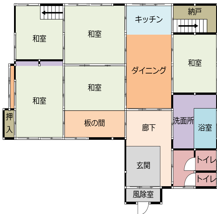
1階平面図
