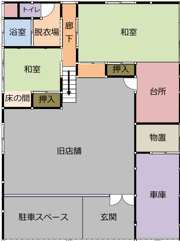
1階平面図
