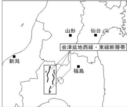
断層位置図
